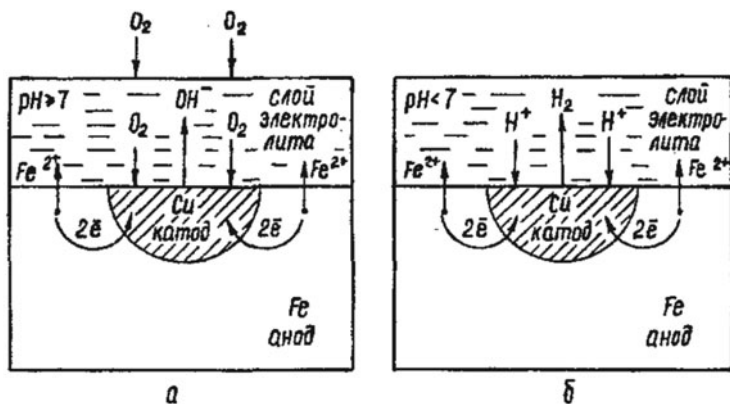
Рис. 26. Схема электрохимической коррозии:
