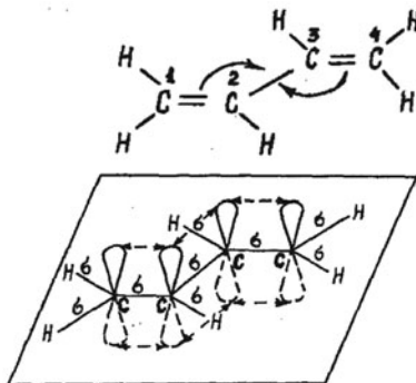
Рис. 30. Схема образования общего \pi -электронного облака в молекуле бутадиена-1,3
