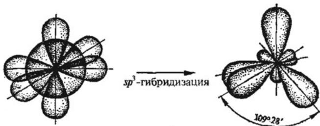
Рис. 13. Образование гибридных sp^3 -орбиталей в атоме углерода
