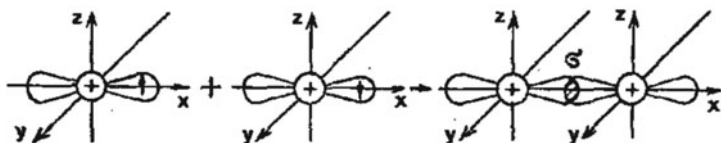
Рис. 4. Схема перекрытия электронных облаков в молекуле хлора
