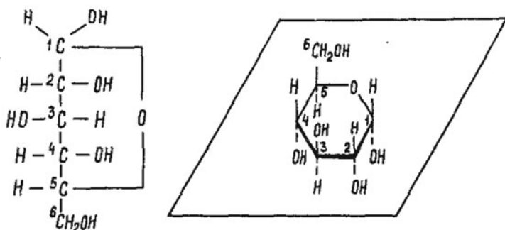
Формула Фишера \leftarrow D-глюкопираноза \rightarrow Формула Хеуэбса
