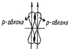
Рис. 5. Образование \pi -связи двумя p -облаками
