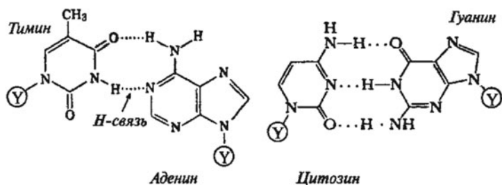
Рис. 38. Образование водородных связей между комплементарными парами оснований
