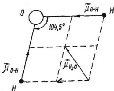
Рис. 8. Определение дипольного момента молекулы воды
