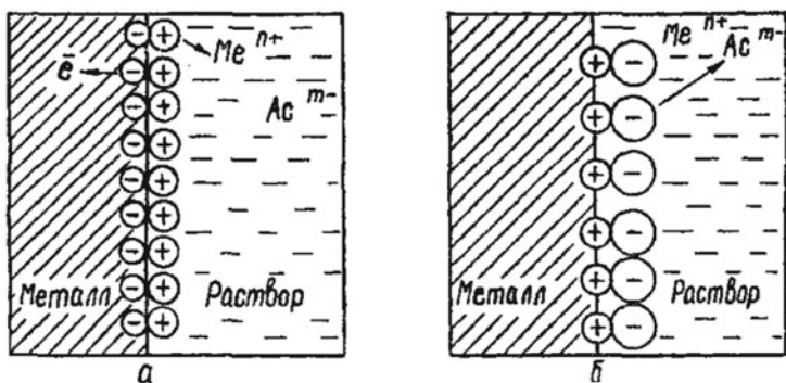
Рис. 23. Образование двойного электрического слоя на границе металл — раствор его соли Me_mAs_n : a — в результате перехода ионов металла в раствор; б — в результате перехода ионов металла из раствора
