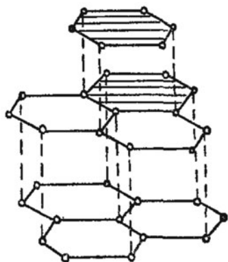
Рис. 29. Строение кристаллической решетки графита
