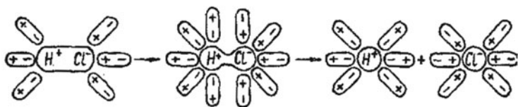
Рис. 22. Схема диссоциации электролита с полярной связью в водном растворе
