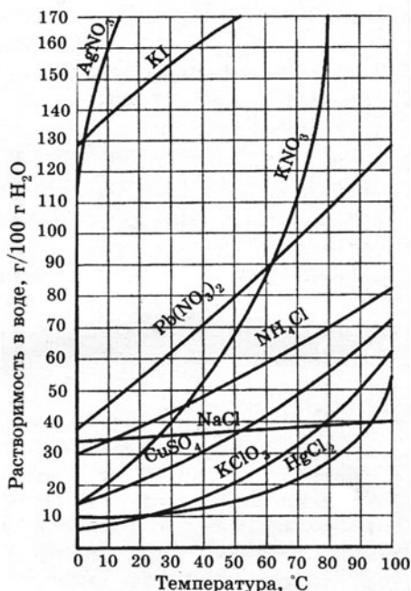
Рис. 20. Кривые растворимости твердых веществ
