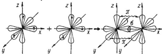
Рис. 6. Схема перекрывания электронных облаков в молекуле азота
