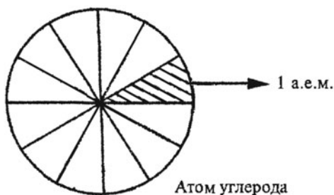
Рис. 1. К определению атомной единицы массы
